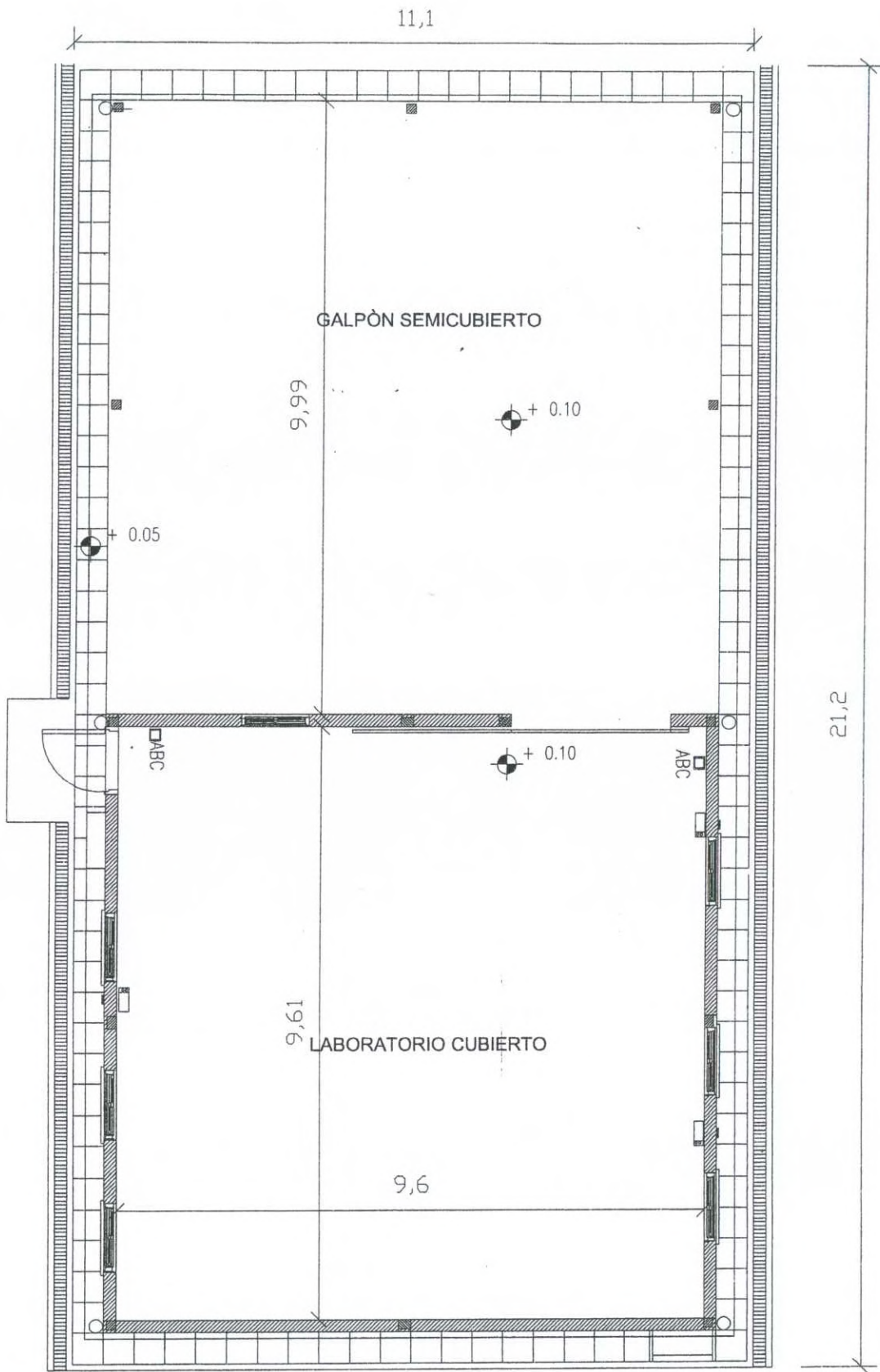
PLANTA GENERAL
